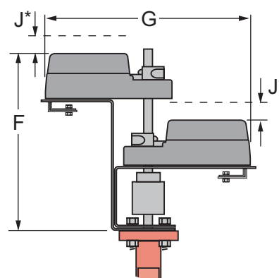
DUAL ACTUATORS
