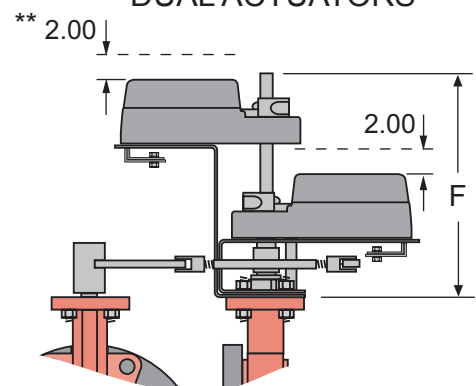
DUAL ACTUATORS
