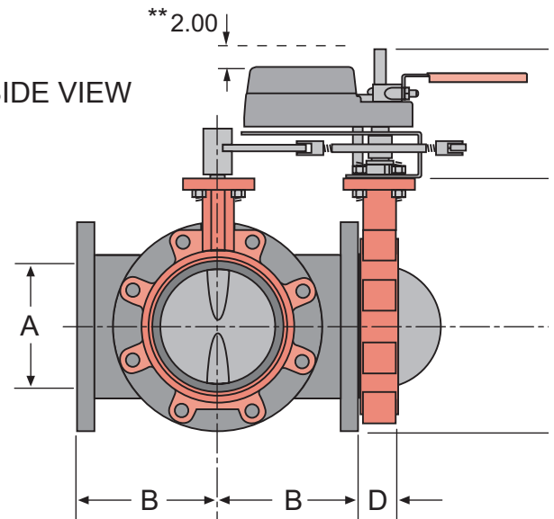
DUAL ACTUATORS
